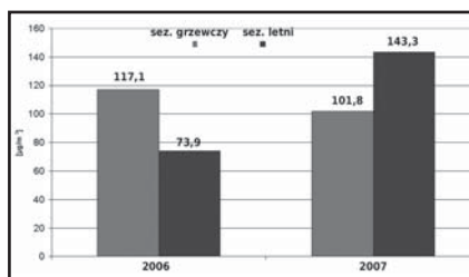
Ryc. 8 Maksymalne stężenia 1 h dwutlenku azotu na stacji ARMAAG w latach 2006-2007.
