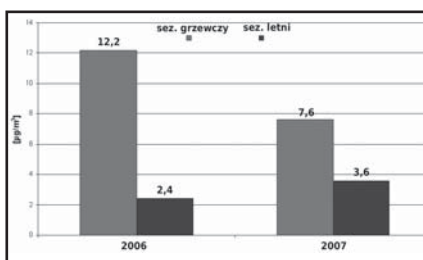
Ryc. 4 Stężenia średniokresowe dwutlenku siarki w sezonie letnim i grzewczym na stacji ARMAAG.
