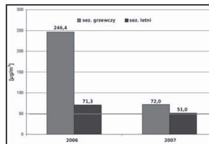
Ryc. 11 Maksymalne wartości stężeń PM10 24 h na stacji ARMAAG, w latach 2006-2007.
