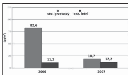
Rys. 5 Maksymalne stężenia średniodobowe dwutlenku siarki na stacji ARMAAG, w latach 2006-2007.
