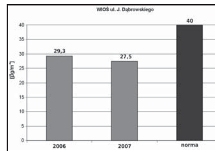
Ryc.10 Zmiany stężeń średniorocznych pyłu zawieszonego PM10 na stanowiskach WIOŚ, w latach 2006-2007.
